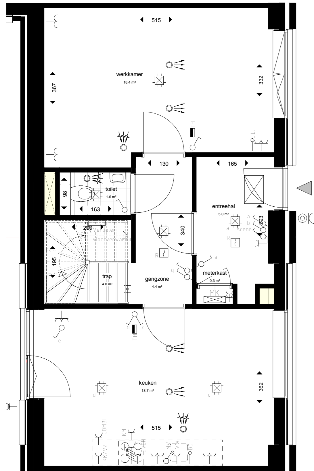
begane grond
