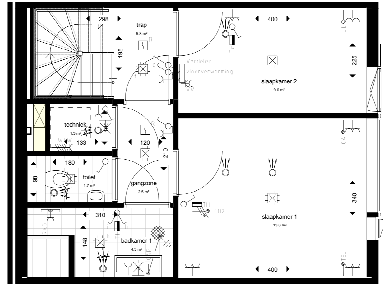
2e verdieping
