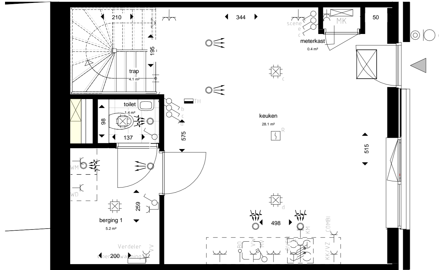
Begane grond
