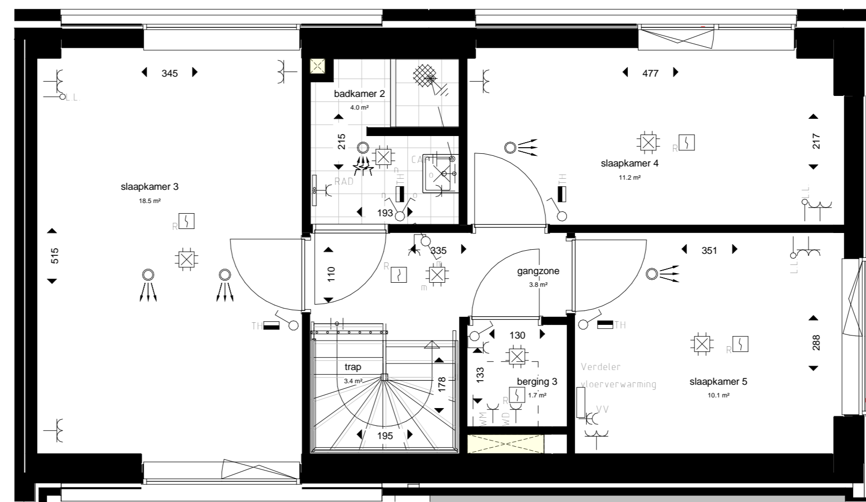
3e verdieping
