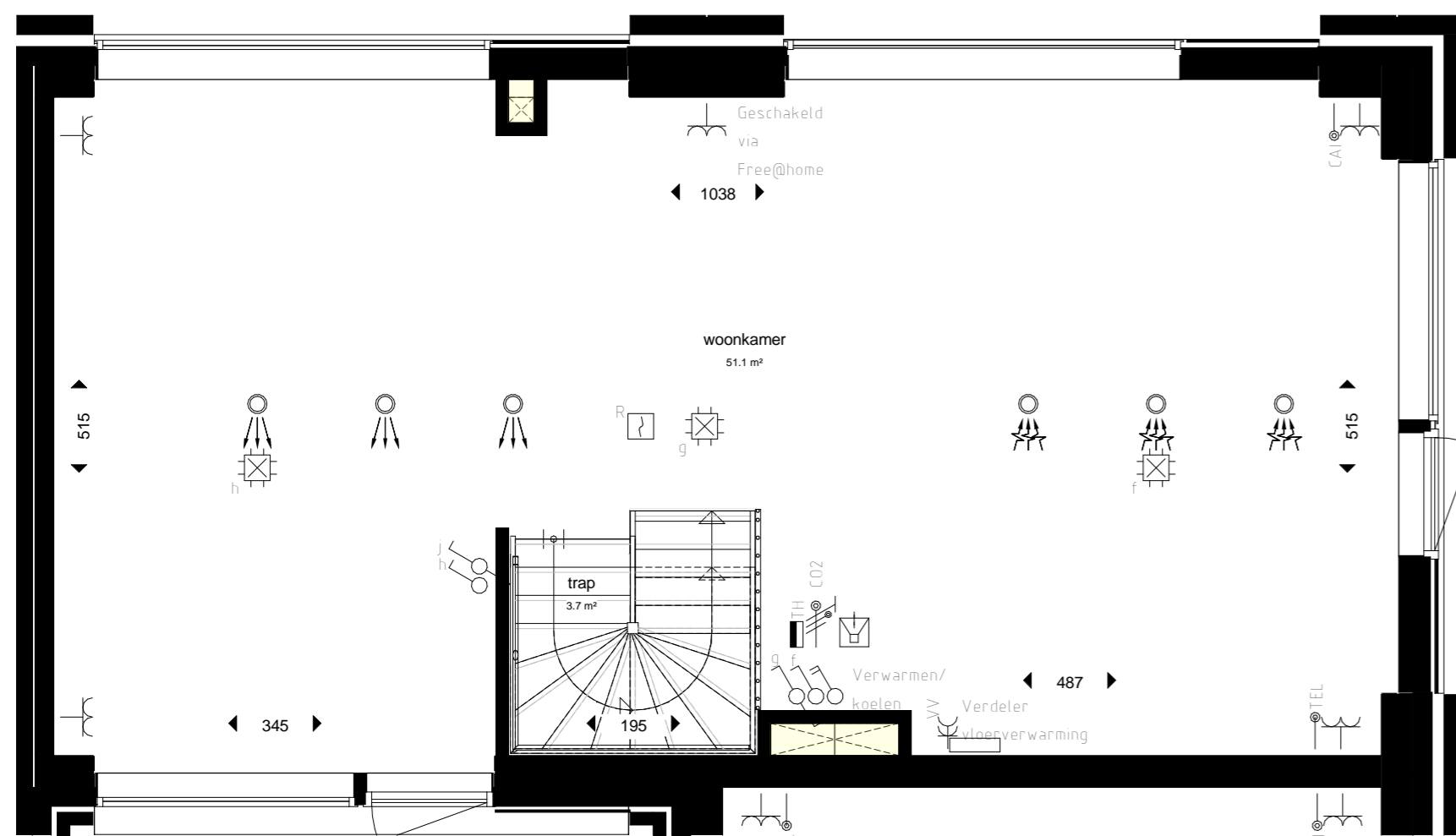
1e verdieping
