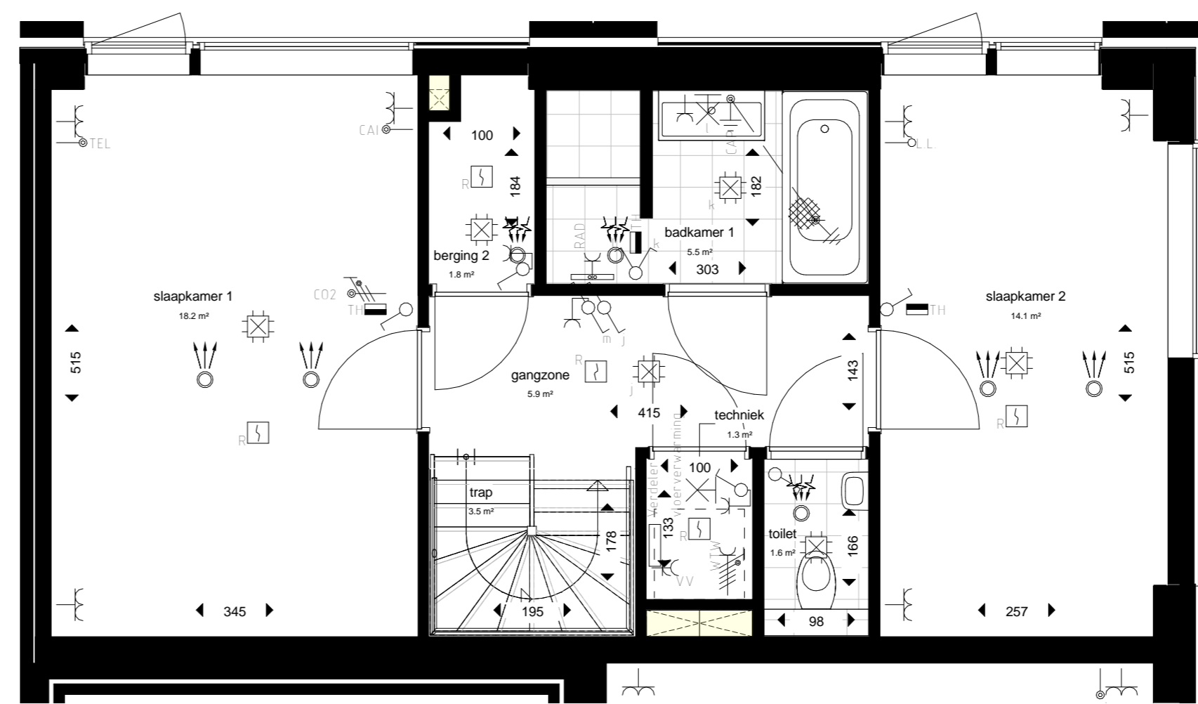
2e verdieping
