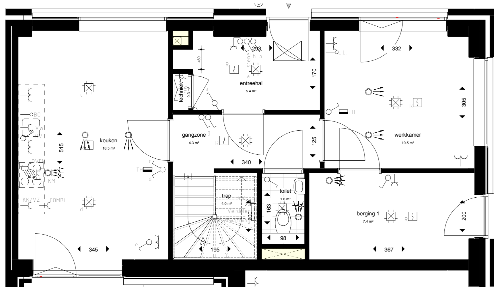
Begane grond
