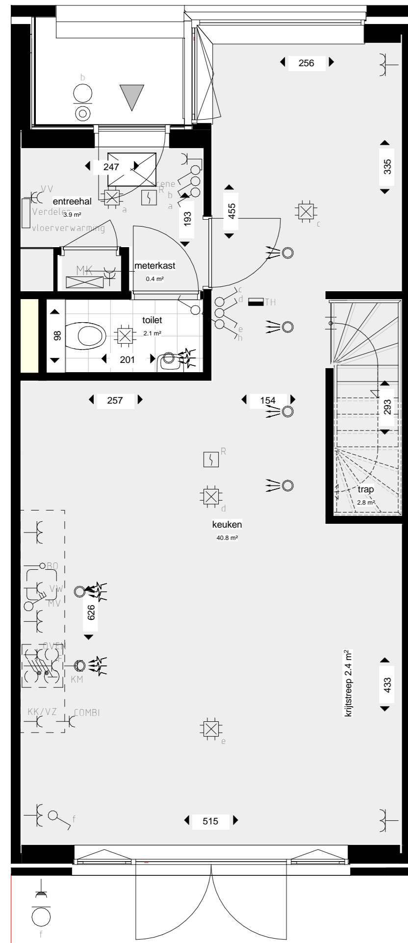
Begane grond
