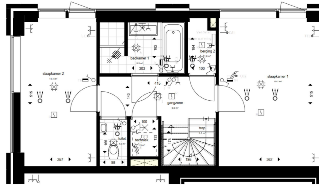
2e verdieping
