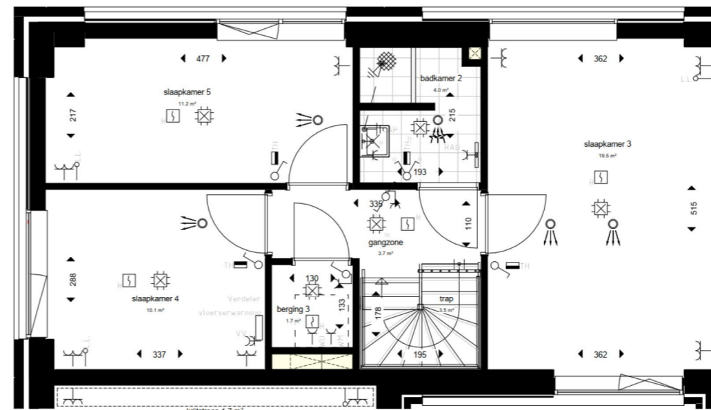
3e verdieping
