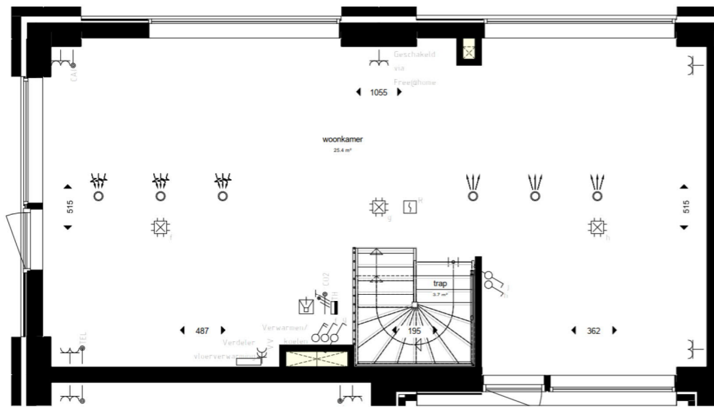
1e verdieping
