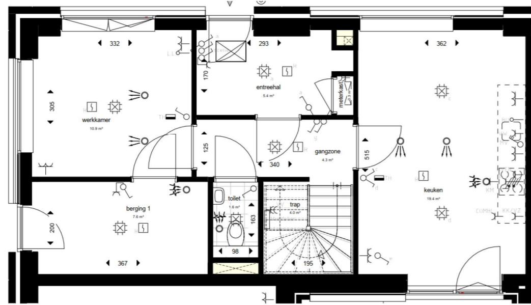
Begane grond
