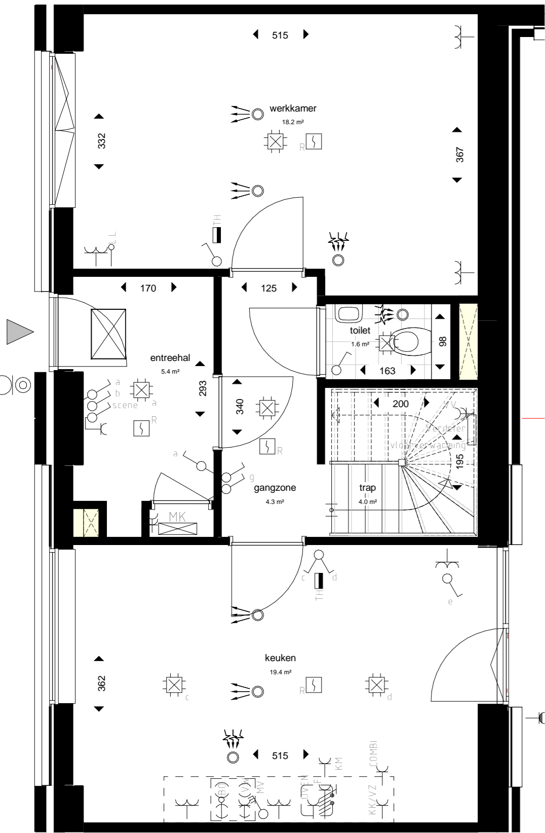
Begane grond
