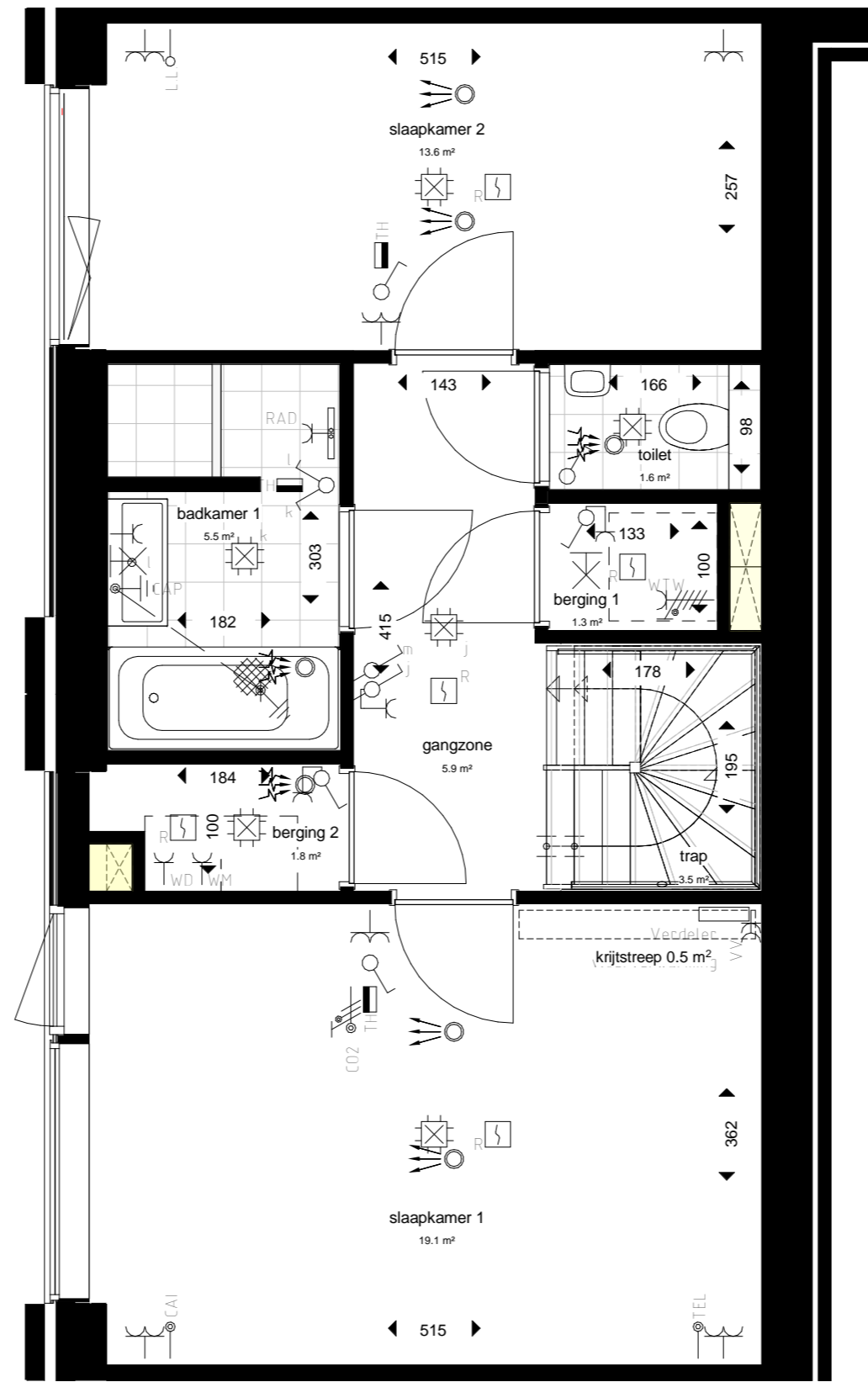
2e verdieping
