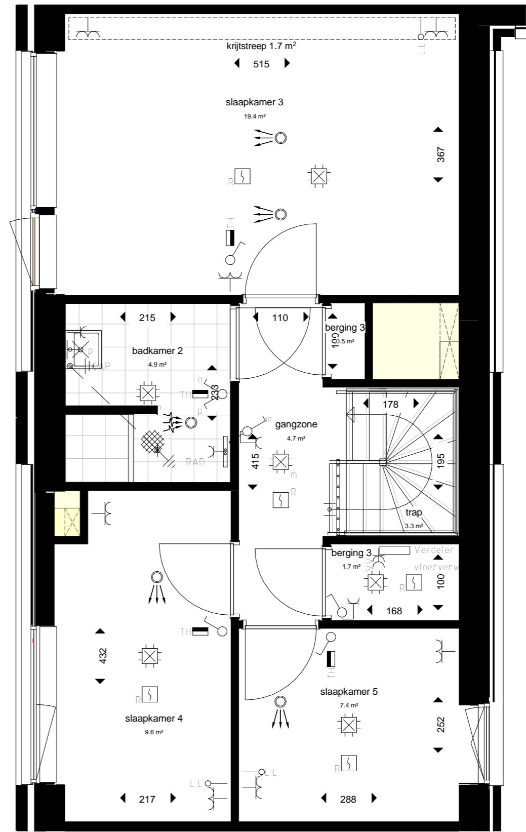
3e verdieping
