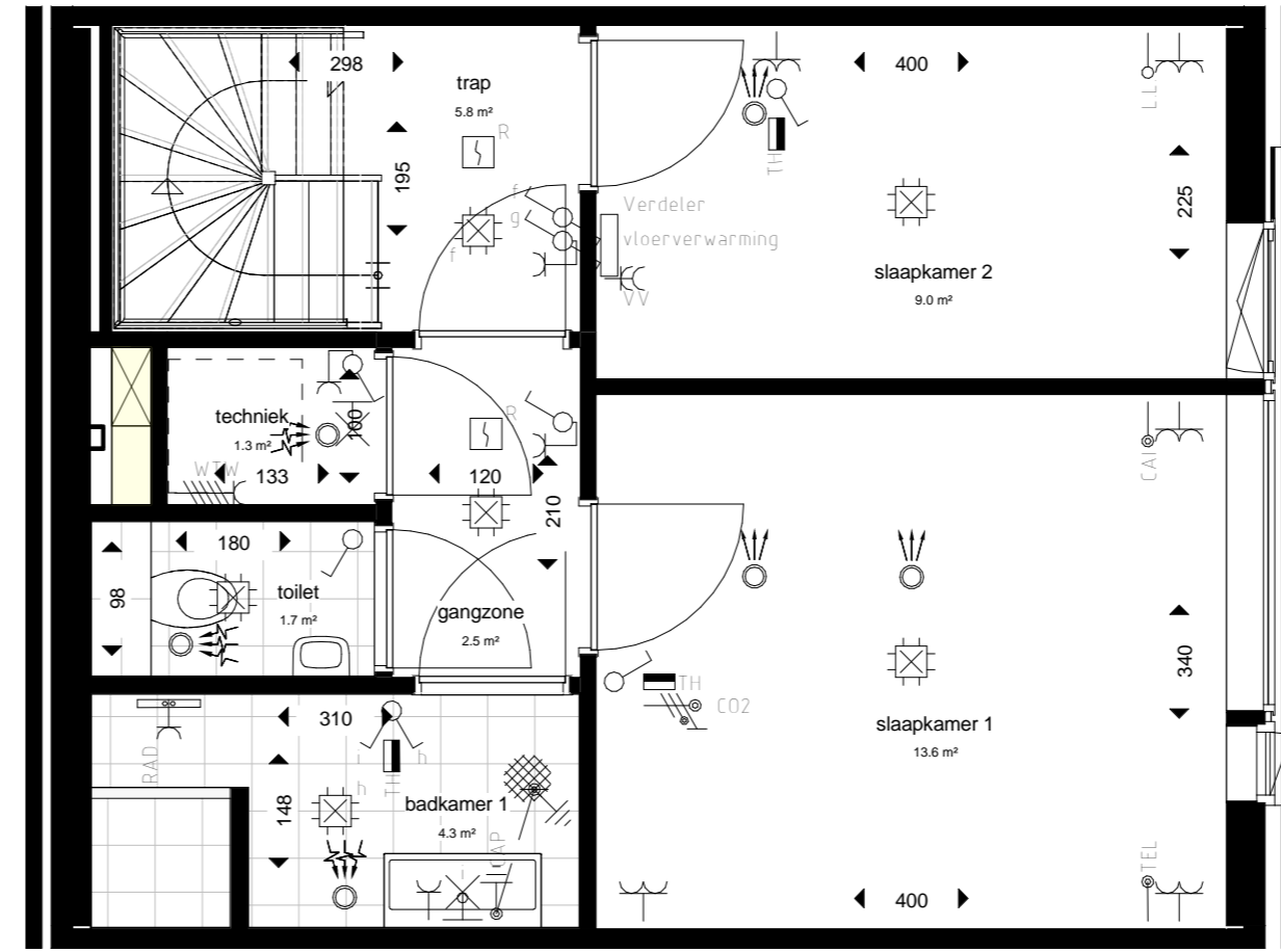
2e verdieping
