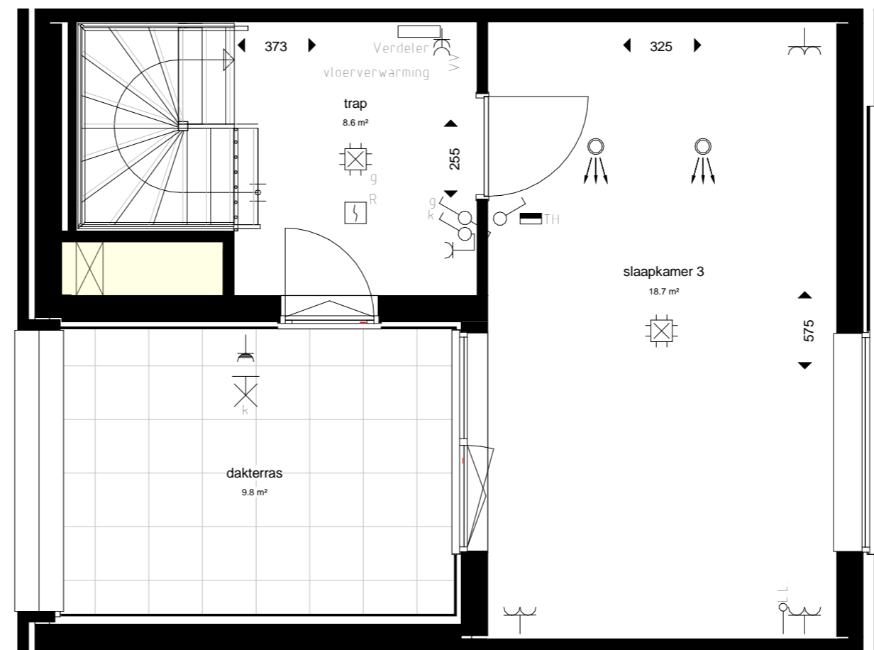
3e verdieping
