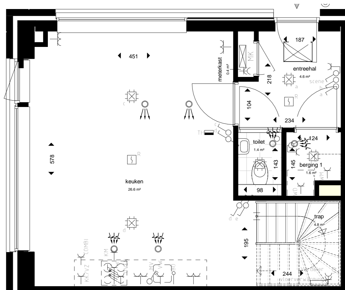
Begane grond
