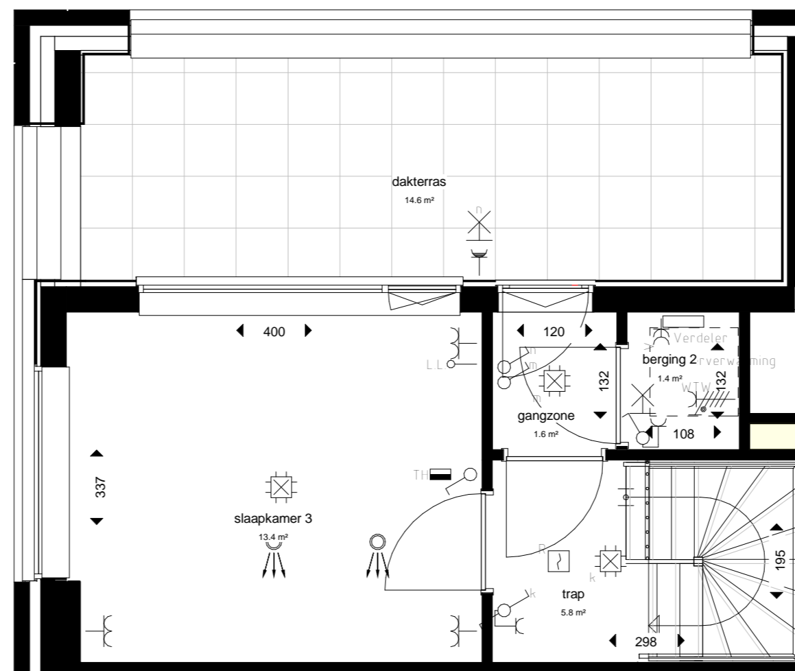
3e verdieping
