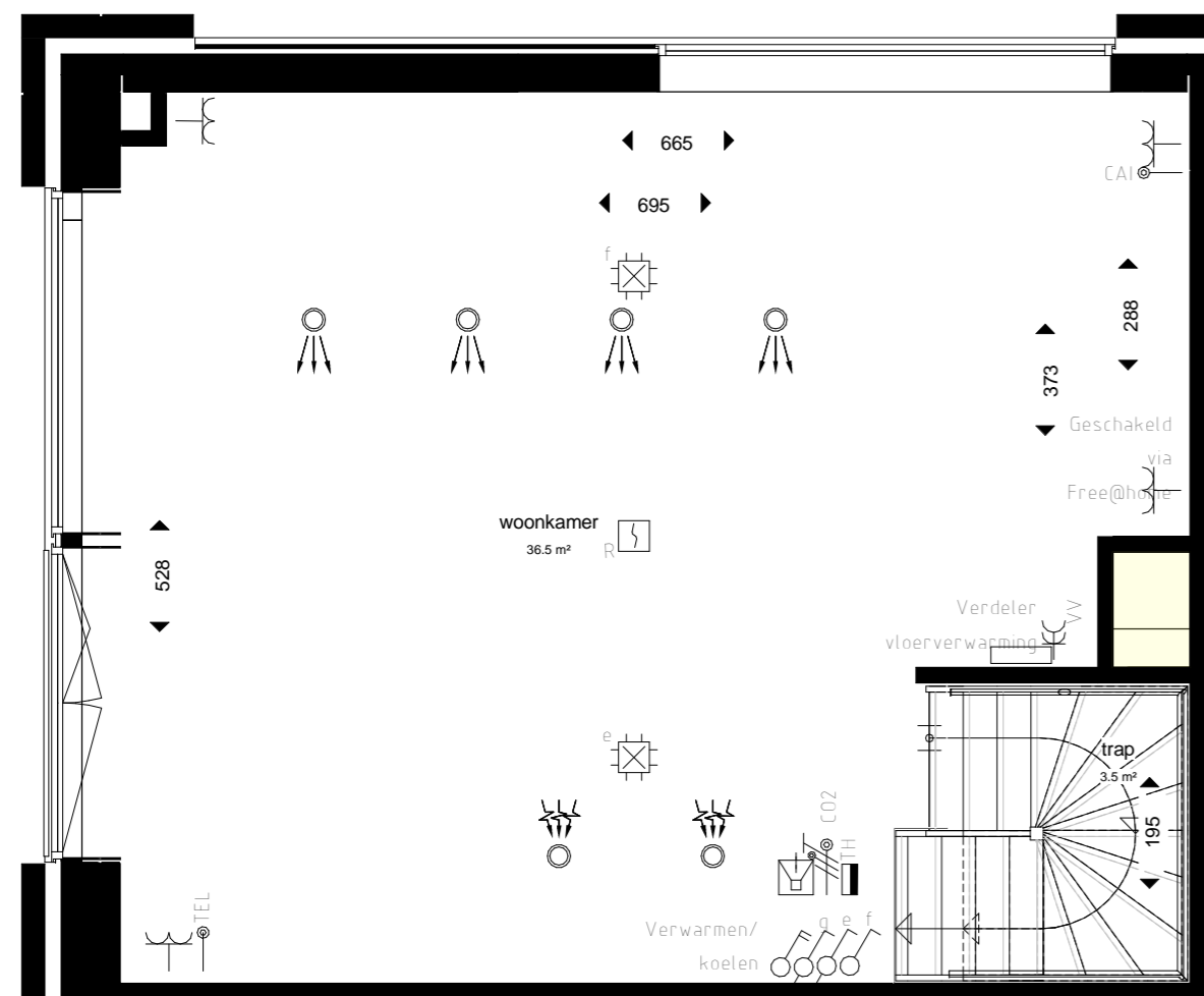
1e verdieping
