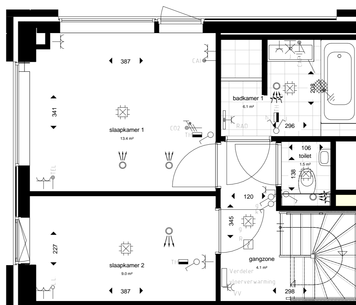
2e verdieping
