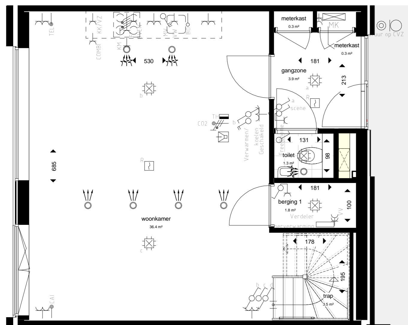
1e verdieping
