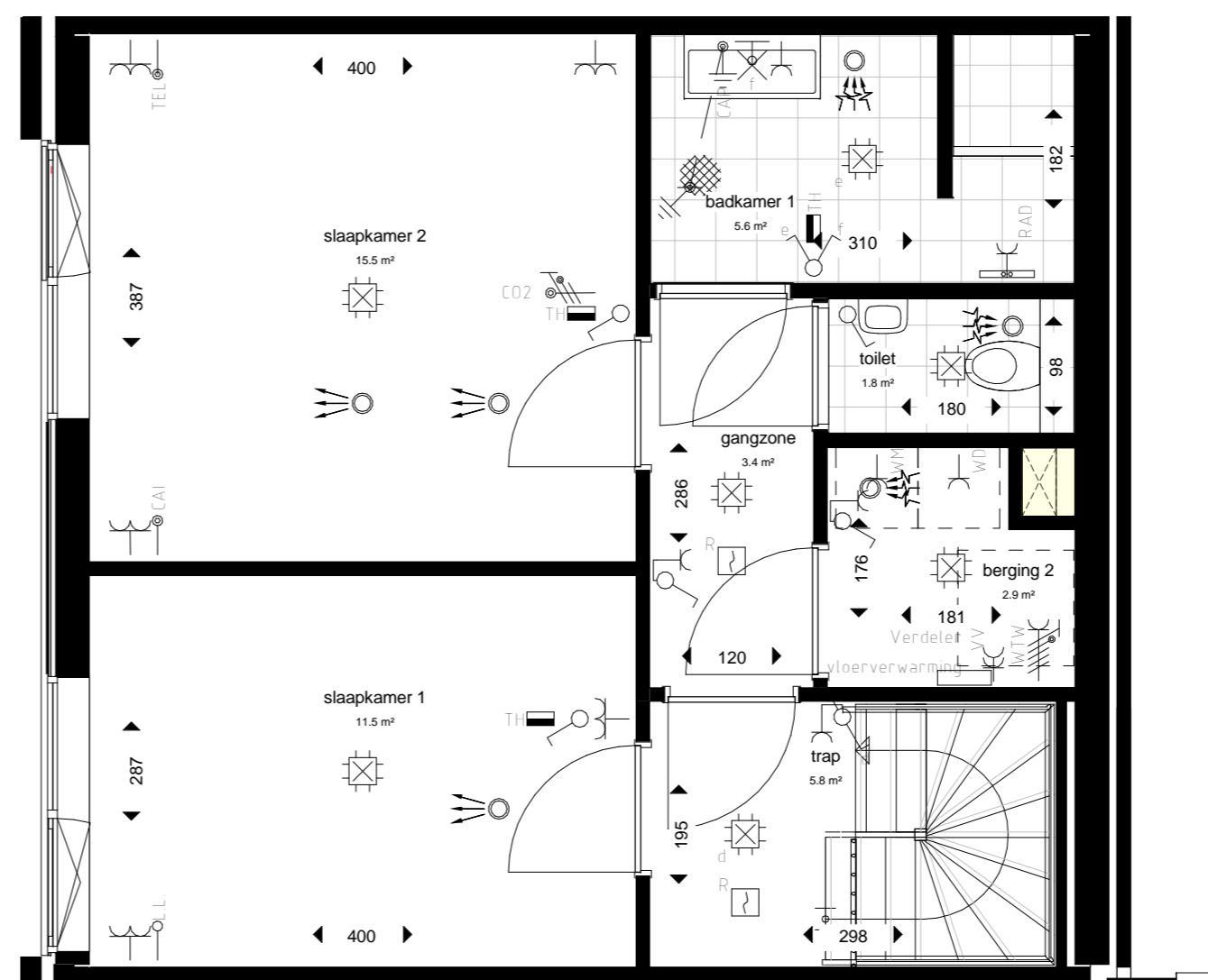
2e verdieping
