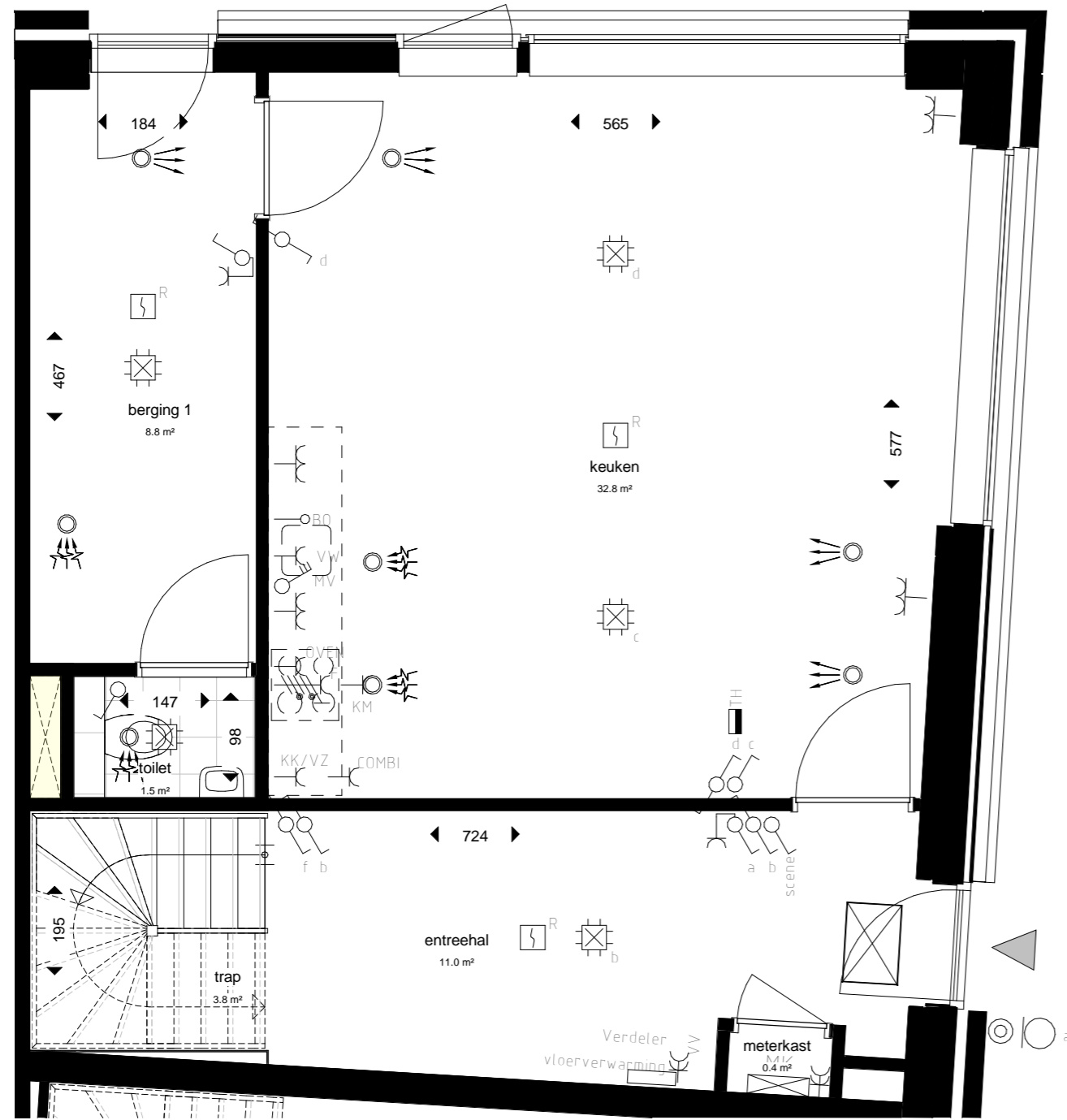
Begane grond
