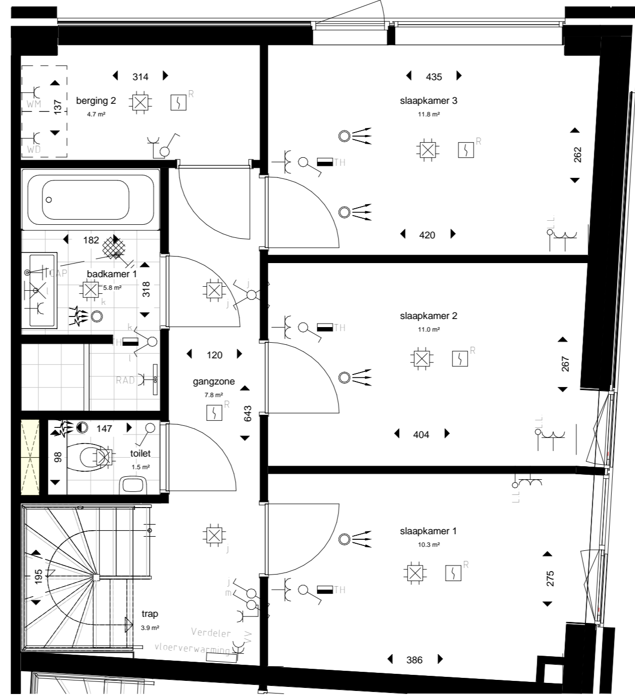
2e verdieping
